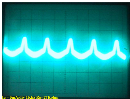
Ig - 5mA/div 1Khz Rg=27Kohm
